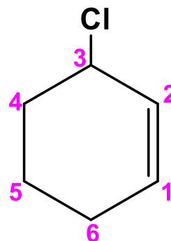
3-klorsikloheksen
