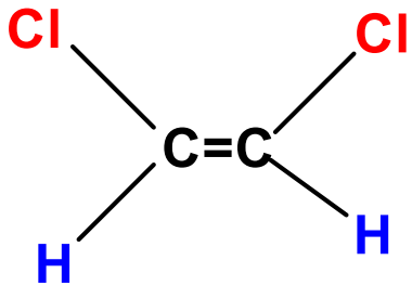
1,2-dikloreten
