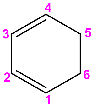
1,3-sikloheksadien
