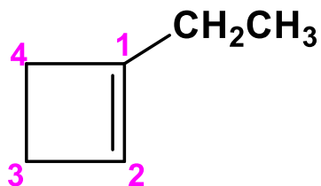
1-etilsiklobuten
