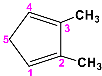
2,3-dimetil-1,3-siklopentadien
