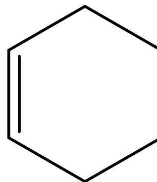
sikloheksen
