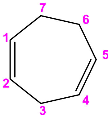
1,4-sikloheptadien
