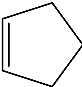
siklopenten
